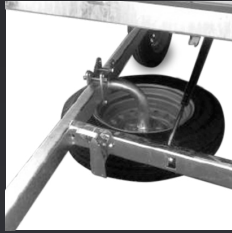
Reservdäckshållare
